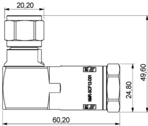
NMR-SCF12-D01_DRW.png
