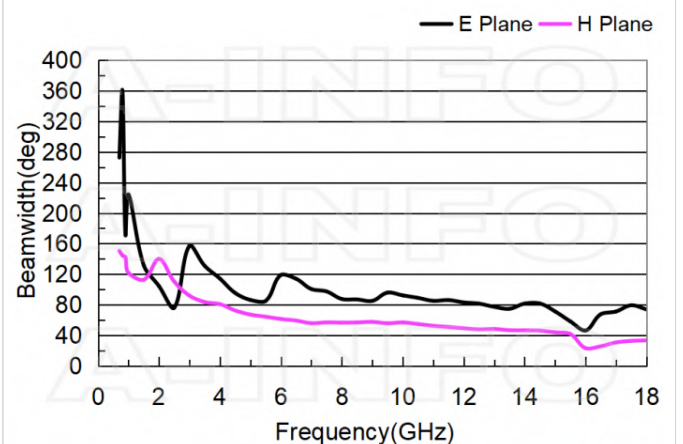
10dB Beamwidth
