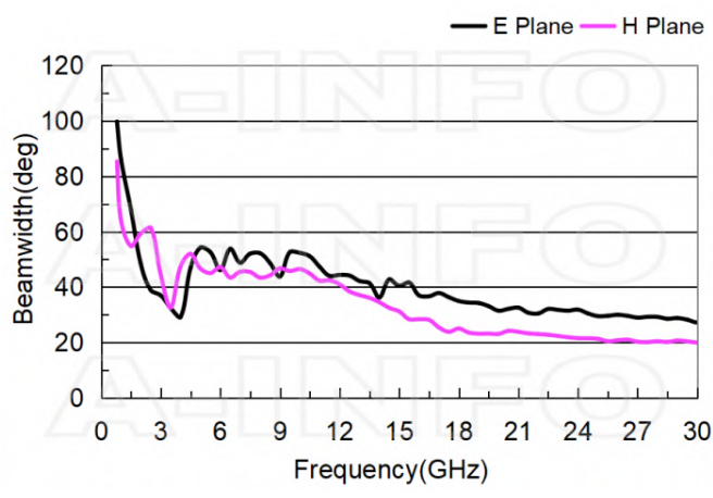
3dB Beamwidth
