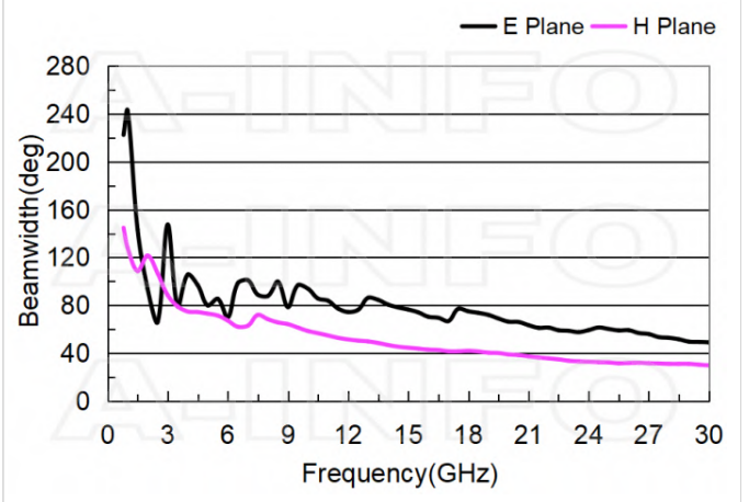
10dB Beamwidth
