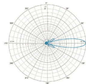
E-Plane | 425 MHz
