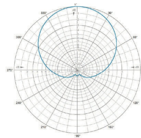
H-Plane | 425 MHz
