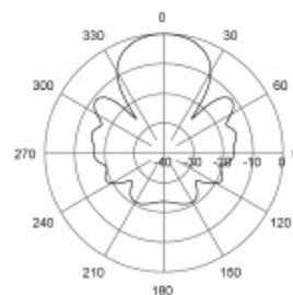
H-Plane | 385 MHz
