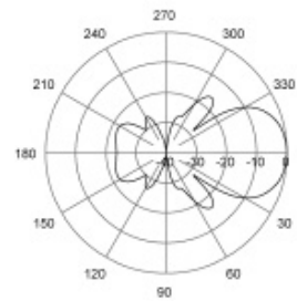
E-Plane | 385 MHz
